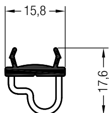
Kältestopp
