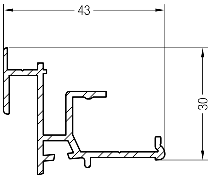
Ausgleichsprofil SYNEGO®
