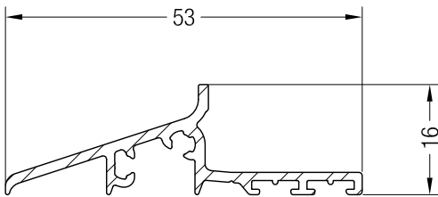
Wetterschenkel SYNEGO®
