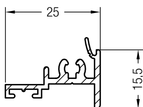
Deckleiste Flügel T SYNEGO®
