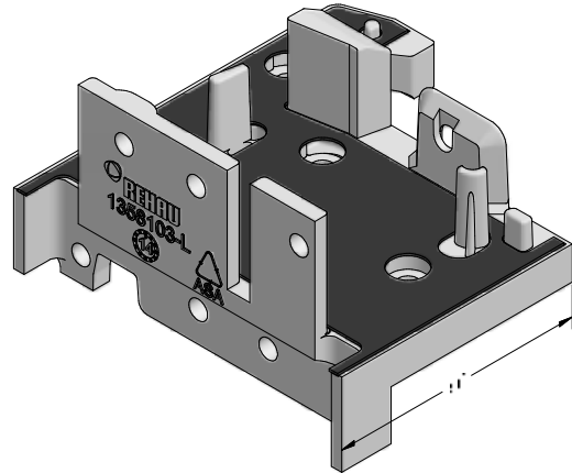
Schwellenhalter Blendrahmen 82 SYNEGO®
